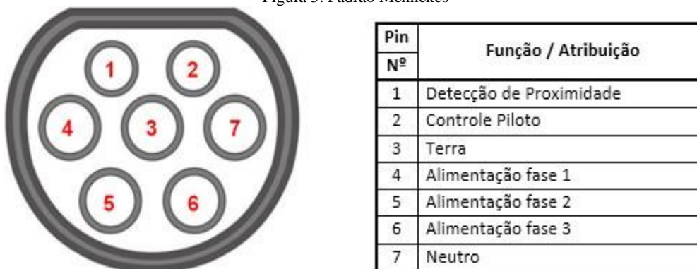
Figura 5. Padrão Mennekes
