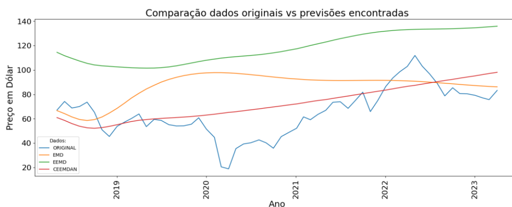
Figura 22. Comparação de dados originais vs previsões encontradas.
