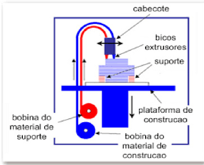
Figura 2: Esquema FDM.
