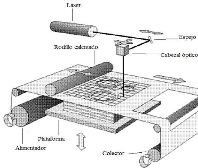
Figura 5: Modelagem de objetos por laminação (LOM).
