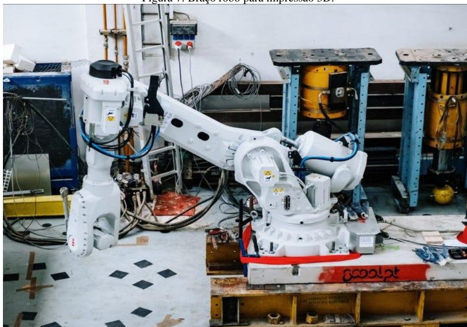
Figura 7: Braço robô para impressão 3D.
