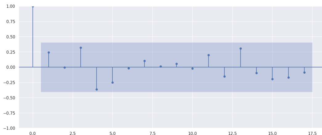
Figura 04. Autocorrelação Parcial
