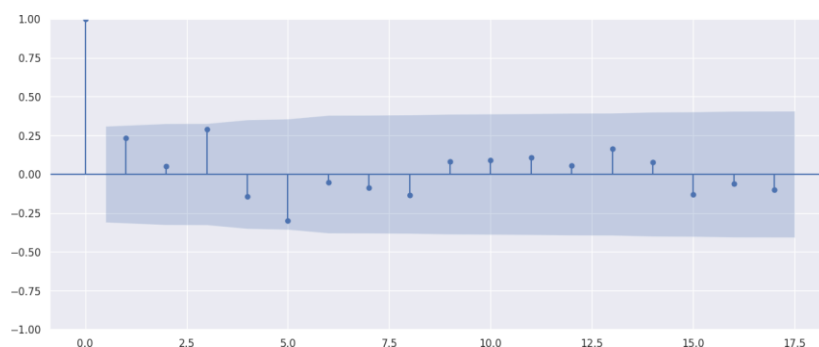
Figura 03. Autocorrelação
