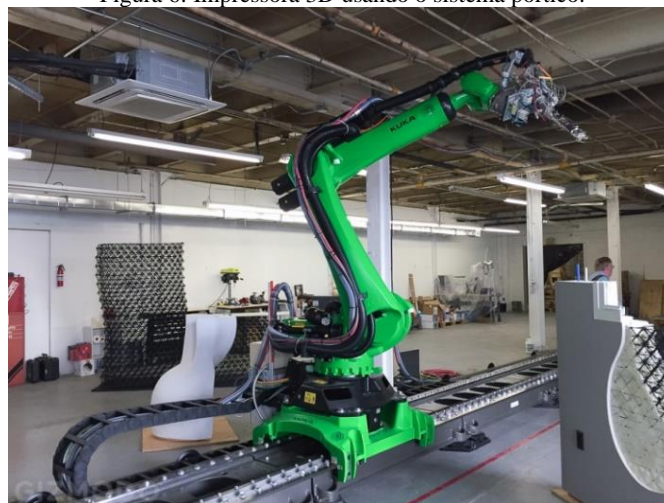
Figura 6: Impressora 3D usando o sistema pórtico.
