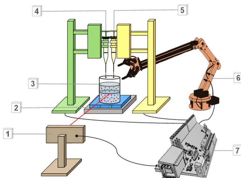
Figura 1: Diagrama esquemático do sistema a ser automatizado do método cloud-point : (1) sensor de turbidez, (2) placa de agitação, (3) vial , (4) seringa para gotejamento de água, (5) seringa para gotejamento de acetonitrila, (6) braço mecânico, e (7) microcontrolador eletrônico do Arduino.
